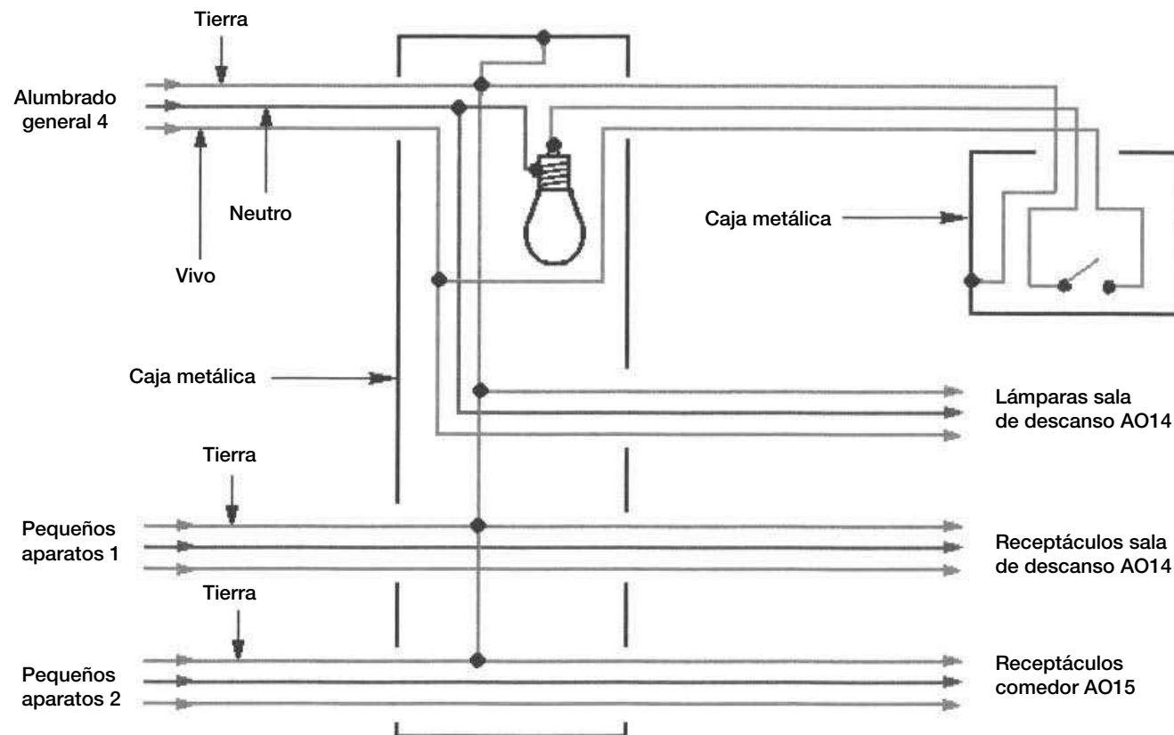
Figura 4.50. Sala de descanso AO14. Circuito de alambrado No. 1
