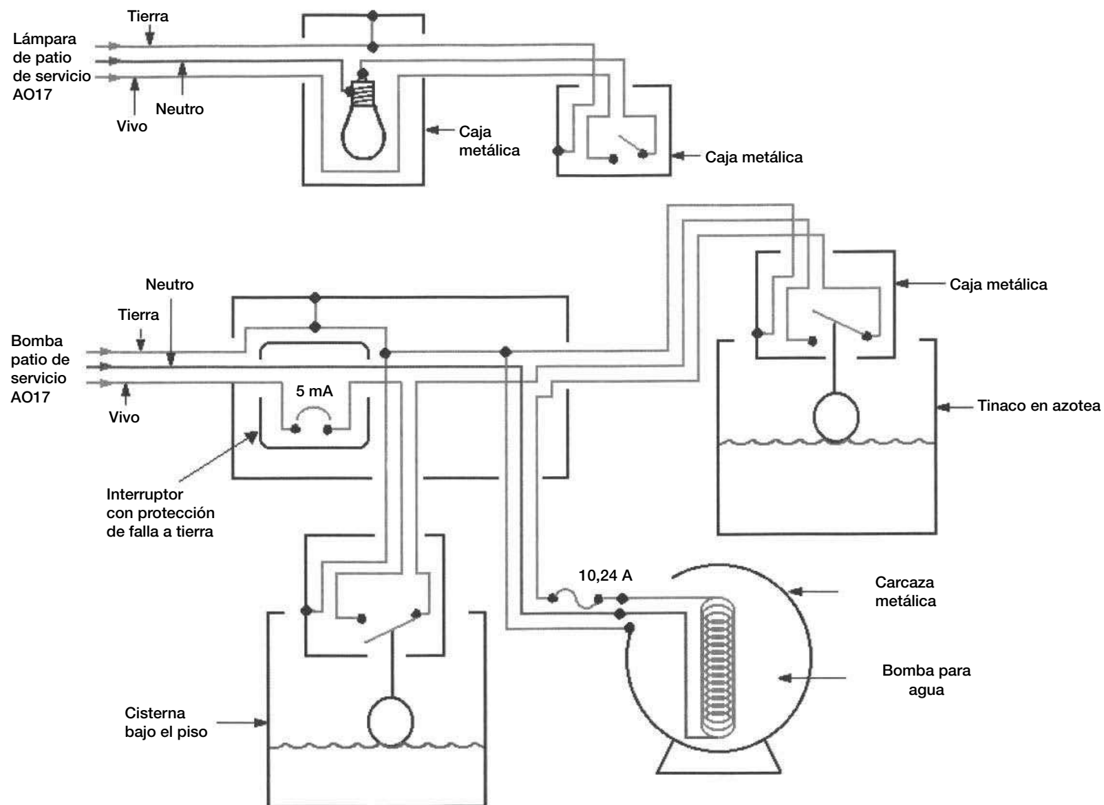
Figura 4.57. Patio de servicio AO17. Circuito de alambroado.
