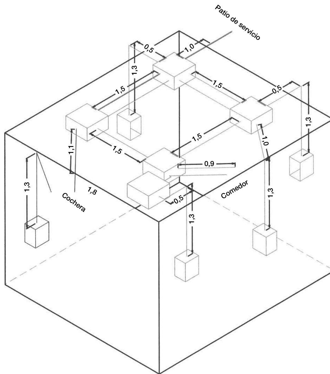
Figura 4.56. Vista en isométrico de tuberías y cajas de conexión. Cocina, área AO16.
