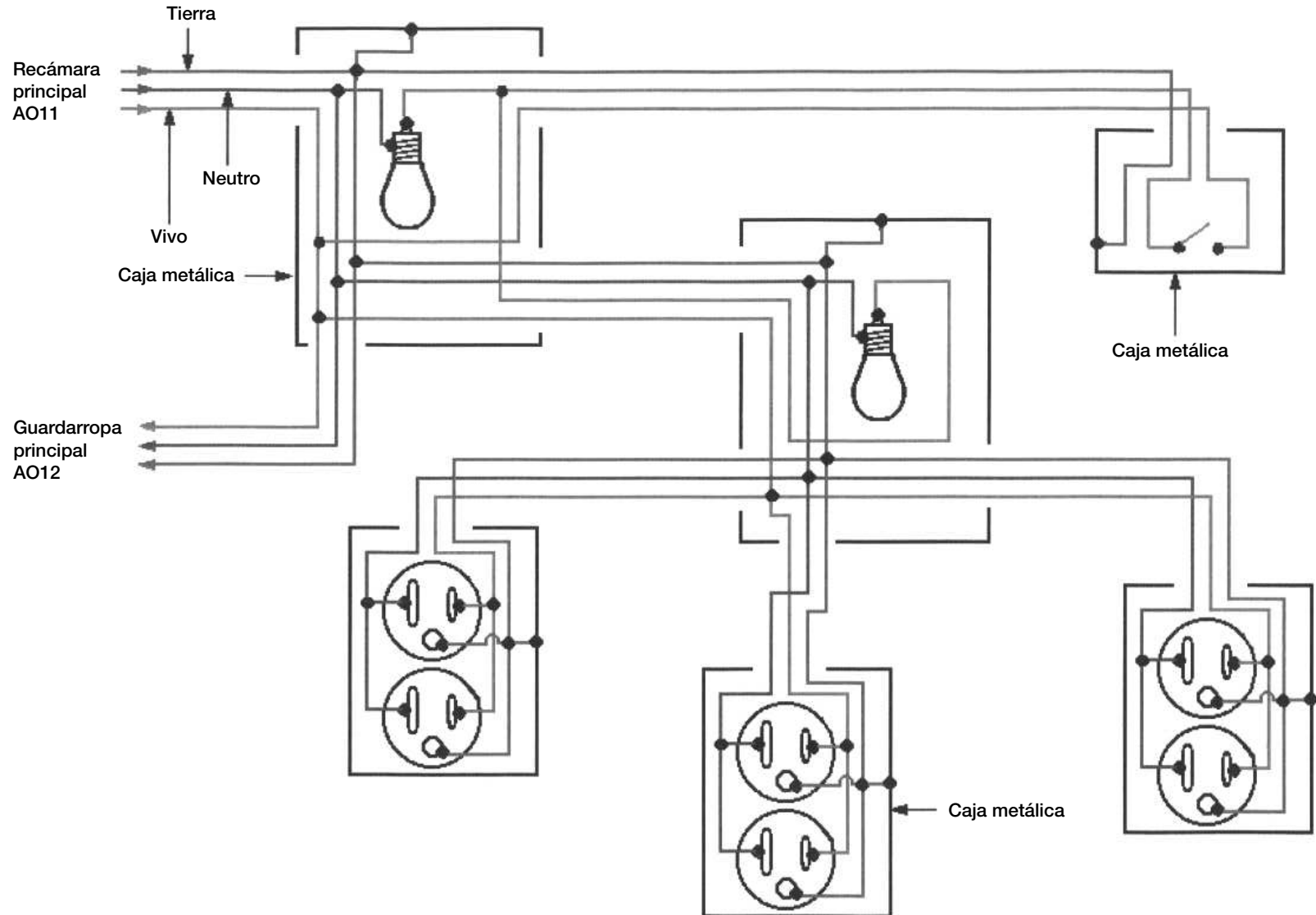
Figura 4.45. Recámara principal, área AO11. Circuito de alambrado
