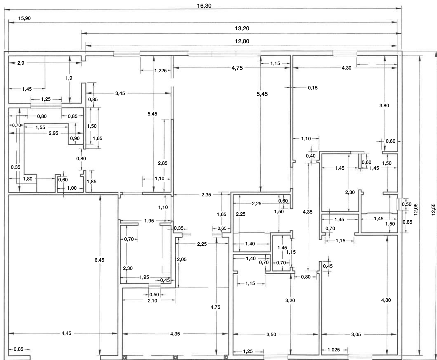
Figura 4.1-A. Dimensiones de una casa habitación.
