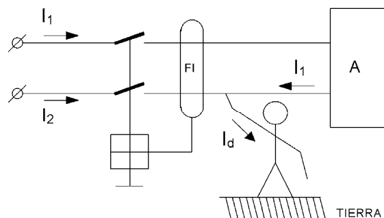
Fig. 3: Actuación de una protección diferencial cuando hay una corriente de defecto (Autor: Fernando Bustillo)
