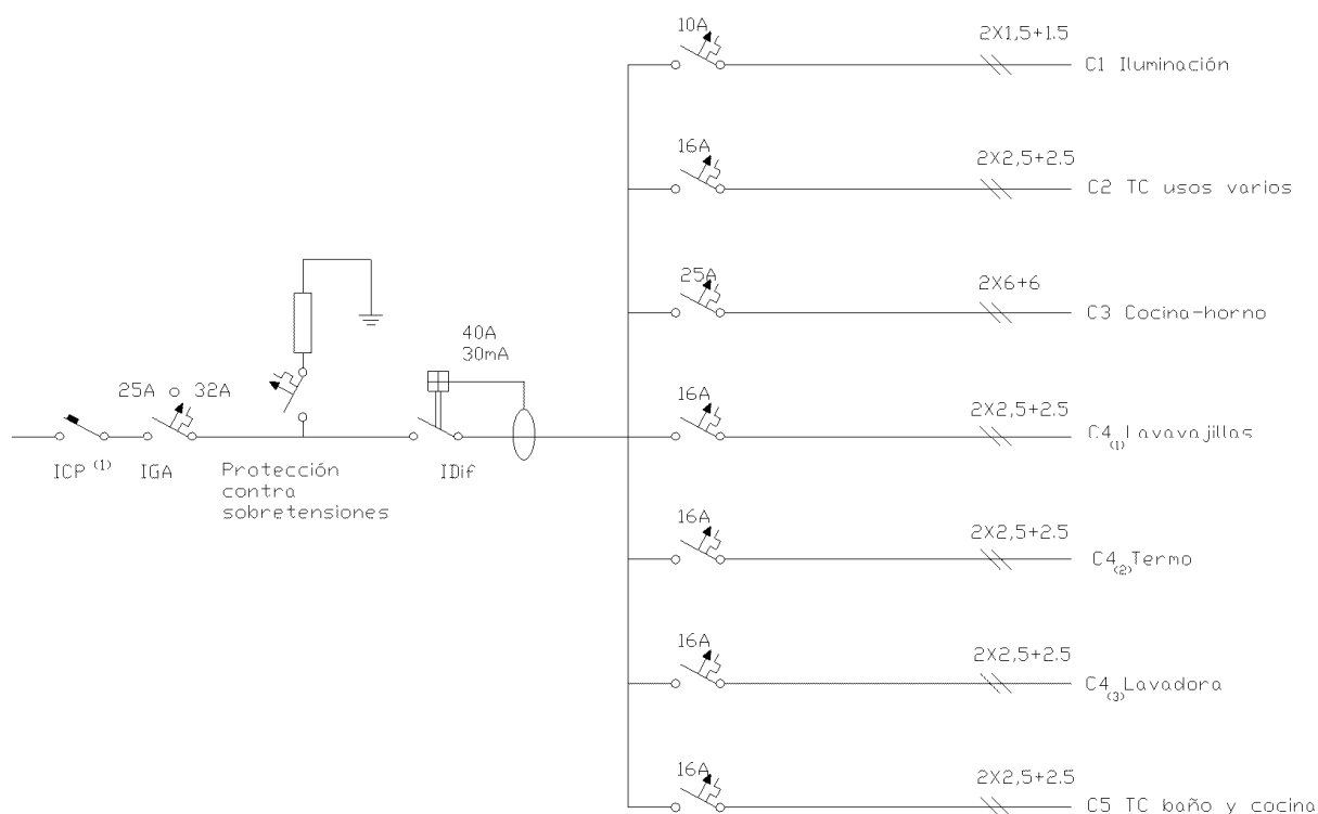
Fig. 19: Ejemplo de esquema unifilar de una vivienda con electrificación básica (Fuente: GUIA-BT-25 [5])
