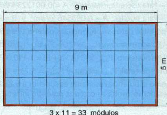
↑ Figura 5.6. Montaje de módulos en posición vertical.
