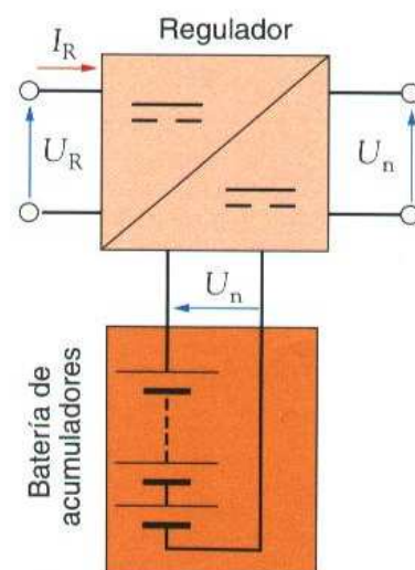
↑ Figura 4.6. Parámetros característicos del regulador de carga.
