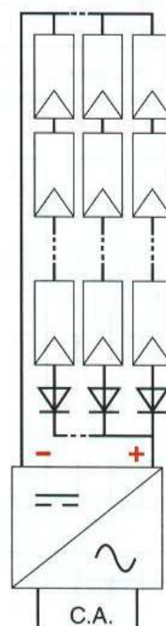
↑ Figura 3.18. Conexionado de módulos a un inversor central.
