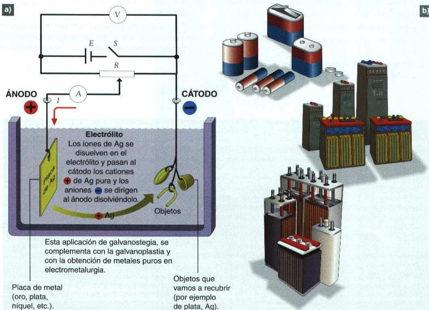
↑ Figura 2.1. Fenómenos electroquímicos: a) Electrólisis b) Pilas primarias y acumuladores.
