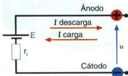
b) Circuito eléctrico
