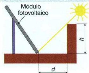
↑ Figura 5.13. Distancia mínima entre módulos y peto perimetral.
