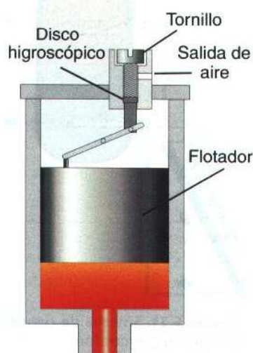
↑ Figura 6.24. Purgador automático.
