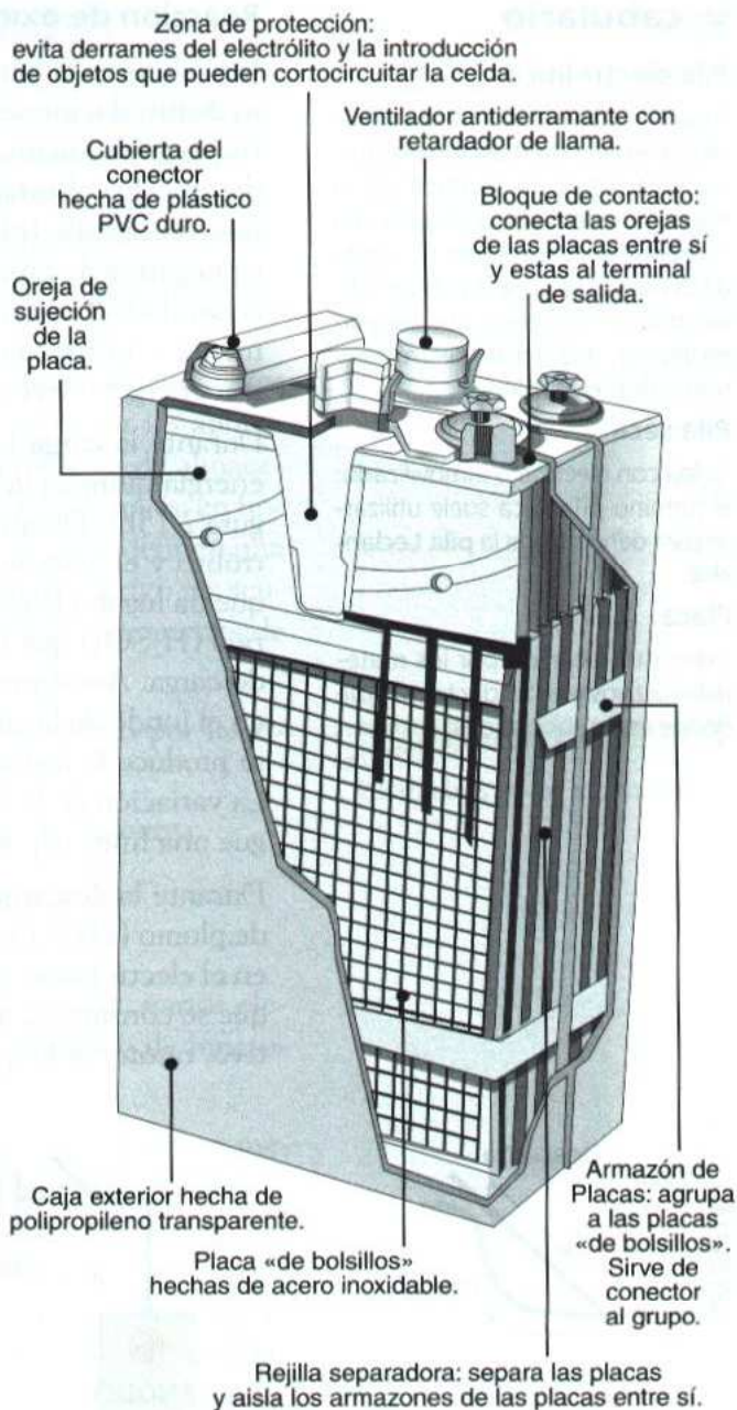
↑ Figura 2.14. Batería de níquel-cadmio (Ni-Cd).
