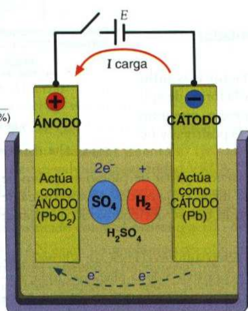
c) Carga
