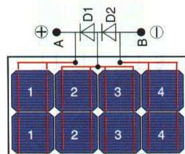
↑ Figura 5.16. Detalle del conexionado de los diodos de paso en un módulo de 32 células.
