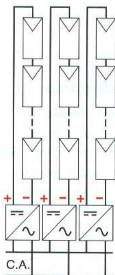
↑ Figura 3.19. Conexión de módulos a inversores de cadena.
