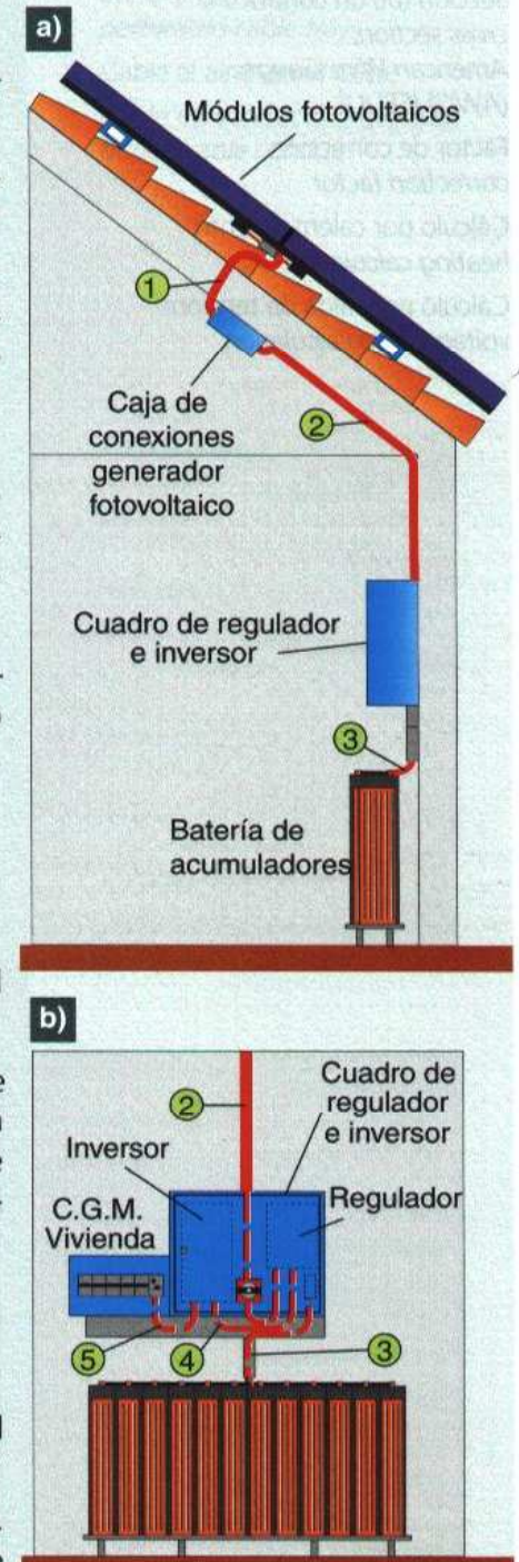
↑ Figura 4.11. Situación de los componentes y canalizaciones eléctricas del proyecto ejemplo.
