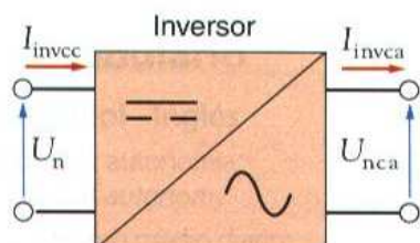
↑ Figura 4.7. Parámetros característicos del inversor.
