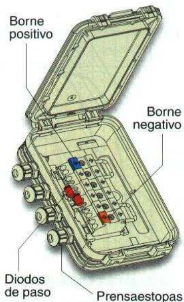
↑ Figura 1.34. Caja de conexiones de un módulo fotovoltaico.
