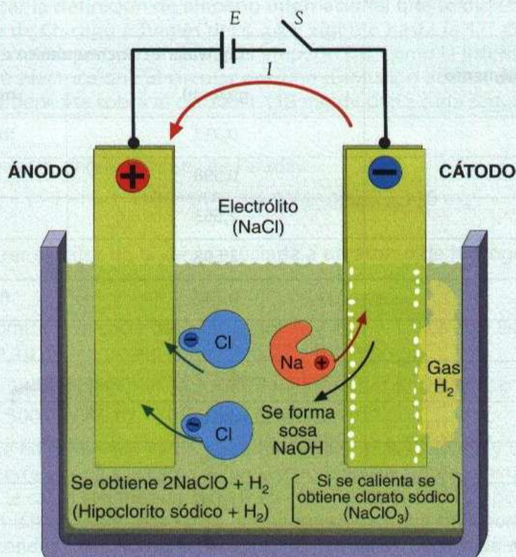
↑ Figura 2.4. Electrólisis de una disolución de cloruro sódico (NaCl).
