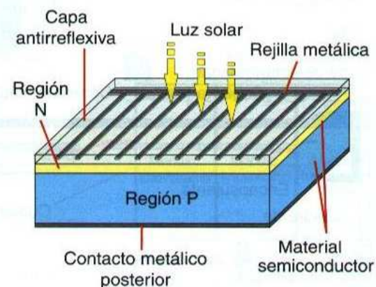
↑ Figura 1.31. Estructura básica de una célula solar.
