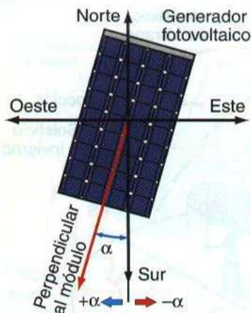
↑ Figura 1.11. Ángulo de acimut ( \alpha ) de un módulo fotovoltaico.
