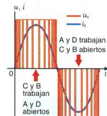
↑ Figura 3.25. Onda PWM producida por un inversor.
