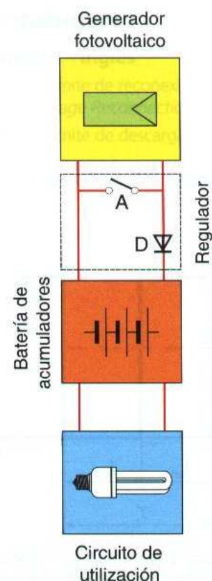
↑ Figura 3.6. Principio de funcionamiento de un regulador paralelo.
