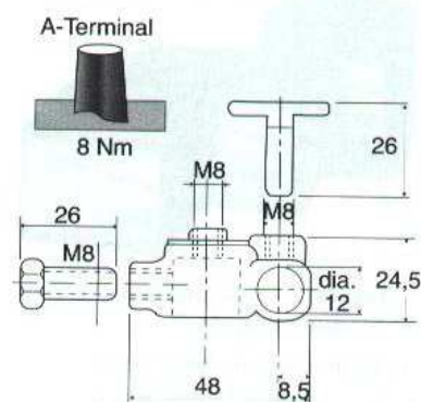
↑ Figura 2.11. Varios terminales de batería. Conjuntos (+) y (-).
