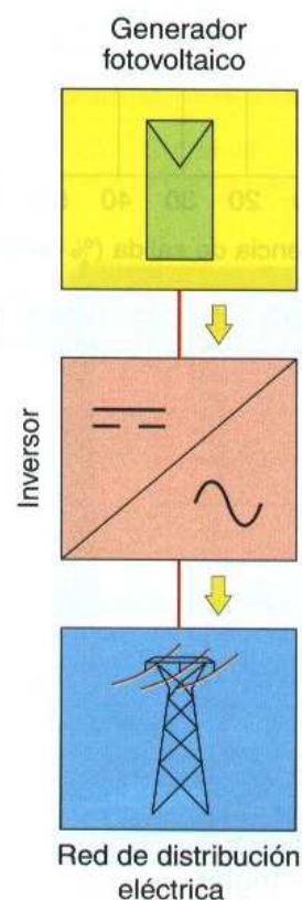
↑ Figura 3.14. Diagrama de bloques de un sistema fotovoltaico conectado a la red.
