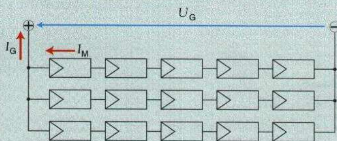
↑ Figura 1.46. Esquema del generador fotovoltaico.
