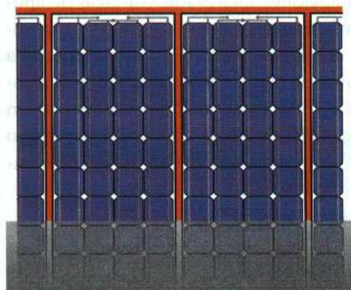
↑ Figura 5.17. Montaje vertical y sombreado inferior.
