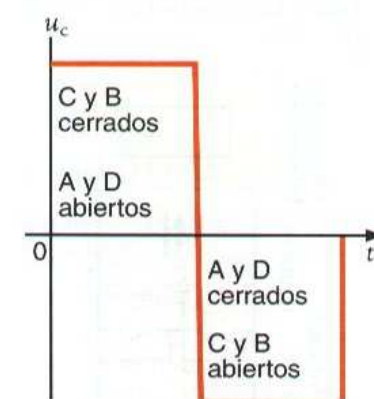
↑ Figura 3.24. Onda cuadrada producida en un inversor elemental.
