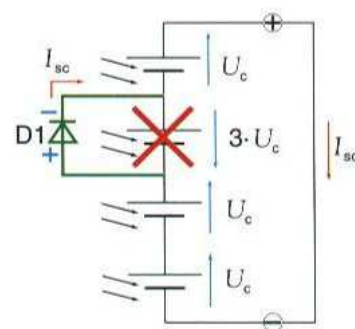
↑ Figura 1.40. Efecto del punto caliente y diodo de paso D1.
