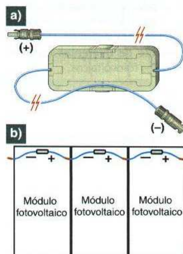
↑ Figura 1.35. Sistema de conexión con conectores. a) Detalle de la caja y los cables. b) Conexionado de módulos en serie.
