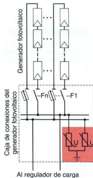
↑ Figura 4.16. Protección contra sobretensiones del generador fotovoltaico.
