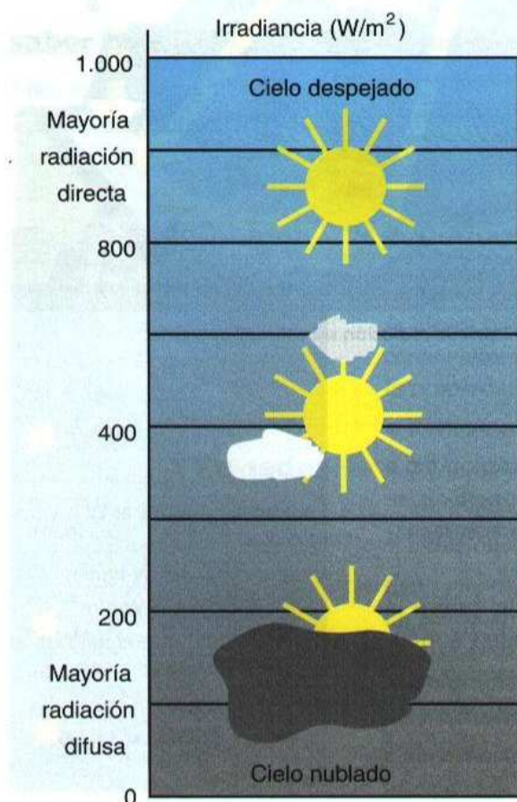
↑ Figura 1.19. Escala de irradiancia en función de la composición de la radiación solar.
