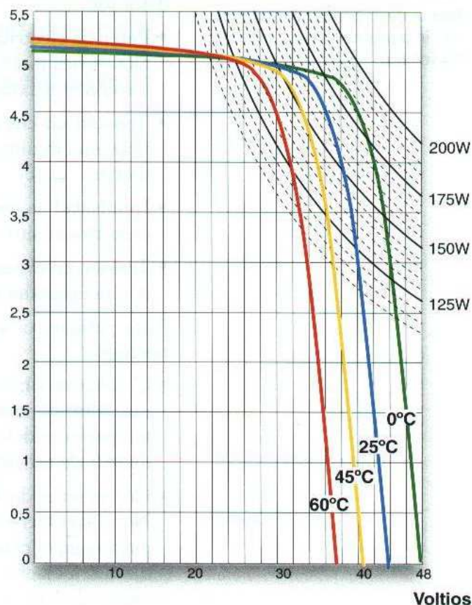
↑ Figura 1.39. Característica i-u con irradiancia de 1000 W/m² en condiciones AM1,5 para diferentes temperaturas de las células.
