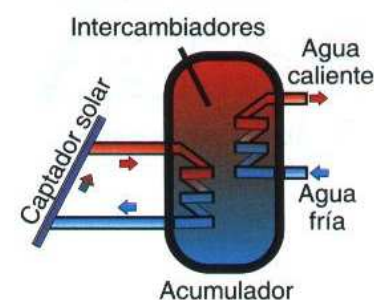
↑ Figura 6.19. Acumulador con dos intercambiadores de calor.
