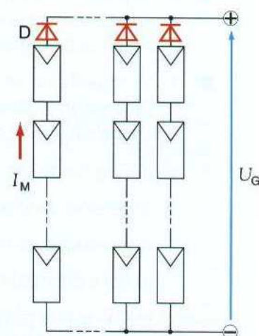
↑ Figura 1.45. Conexión de diodos de bloqueo en las ramas de un generador fotovoltaico.
