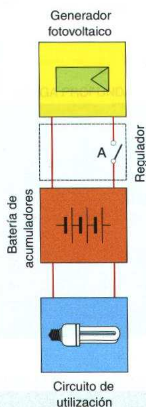
↑ Figura 3.5. Principio de funcionamiento de un regulador serie.
