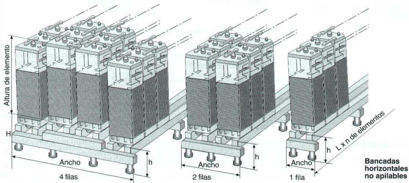
↑ Figura 2.20. Bancada de baterías.
