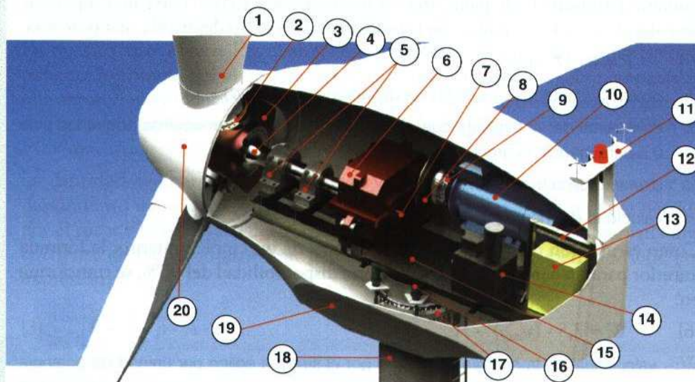
↑ Figura 6.9. Aerogenerador de eje horizontal (Electria Wind).
