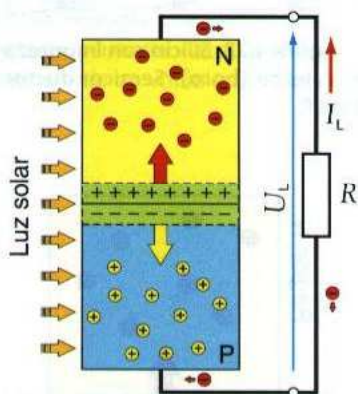
↑ Figura 1.26. Célula solar conectada a un receptor.
