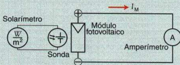
↑ Figura 1.53. Esquema para comprobar la corriente de cortocircuito de un módulo fotovoltaico.
