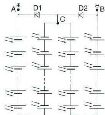
↑ Figura 1.37. Esquema eléctrico de un módulo fotovoltaico con sus células en serie (véase epígrafe 9.6).
