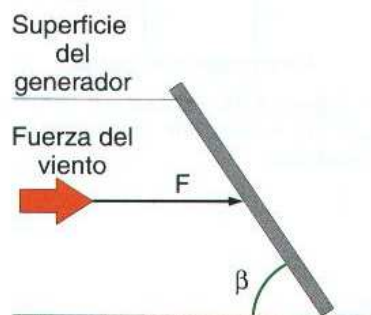
↑ Figura 4.18. Fuerza del viento sobre el plano posterior de un generador fotovoltaico.
