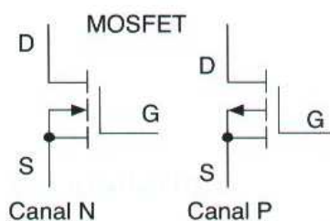
Símbolos eléctricos de transistores MOSFET.
