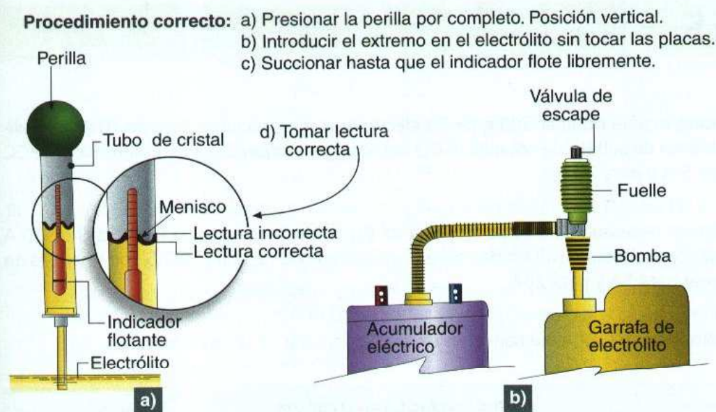
↑ Figura 2.22. Comprobación del electrolito: a) lectura del densímetro; b) utilización de un sifón de llenado.
