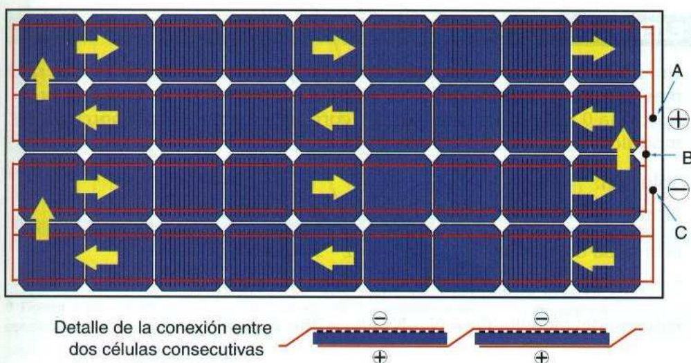
↑ Figura 1.36. Conexionado de las células de un módulo fotovoltaico de silicio monocristalino. Se indica el sentido de circulación de la corriente.
