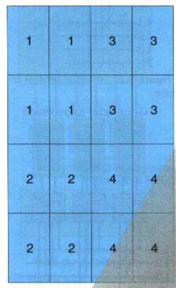
↑ Figura 5.20. Sombreado lateral sobre un generador fotovoltaico.
