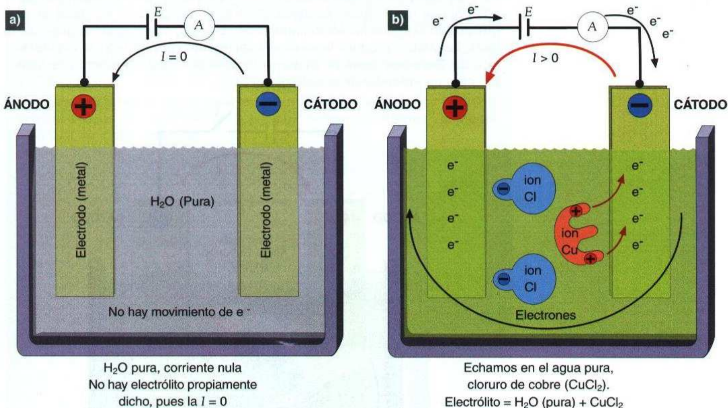
↑ Figura 2.2. Teoría electrónica de la electrólisis: a) No hay disociación electrónica del agua pura. b) Disociación de la molécula de cloruro de cobre ( \text{CuCl}_2 ).
