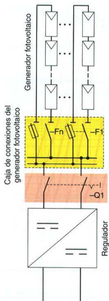
↑ Figura 4.14. Elementos de maniobra y protección del generador fotovoltaico.
