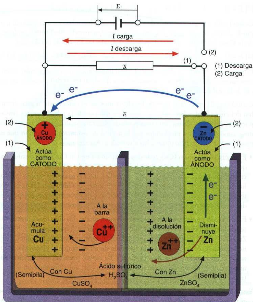
↑ Figura 2.8. Pila Daniell como elemento galvánico reversible: DESCARGA /CARGA.
