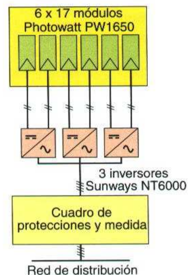
↑ Figura 5.25. Esquema unifilar del generador fotovoltaico del ejemplo (se omiten los aparatos de maniobra y protección).
